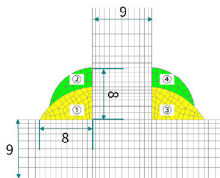
本来の溶接
