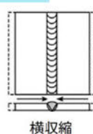
横収縮
